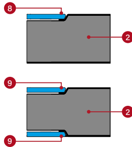
Panou fățuit cu suprafața canatului, realizat din sticlă neagră vopsită.
