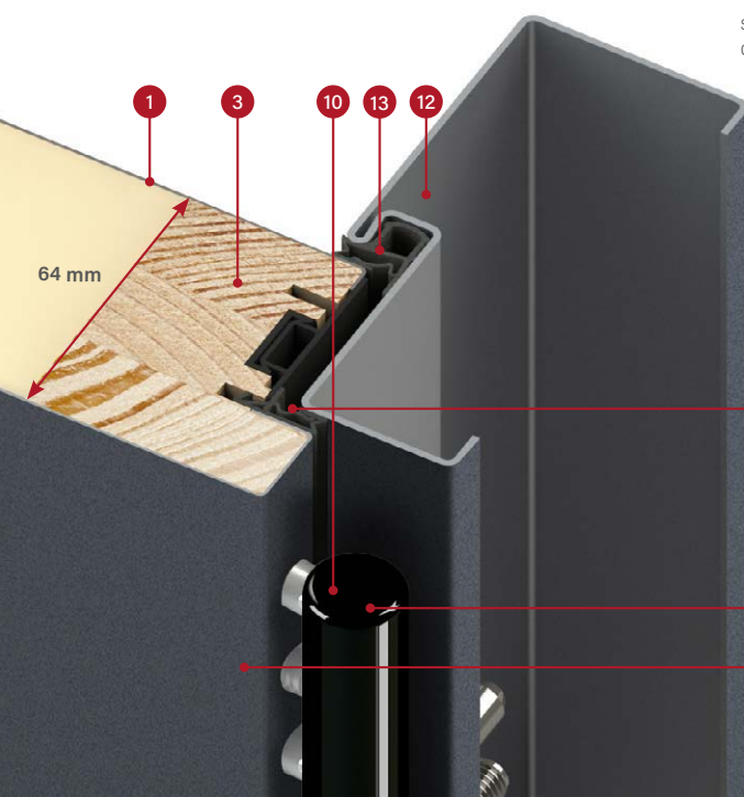
secțiunea transversală a tocului din oțel pentru canatul THERMO 64
