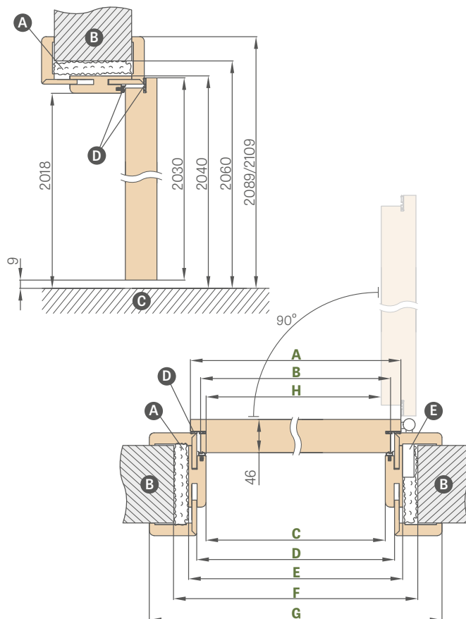
SCHEMA TOC REGLABIL HERSE SET
